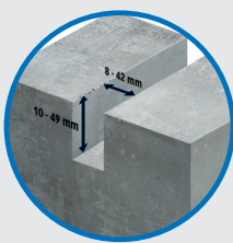
● LARGEUR RÉGLABLE 8-42 MM PROFONDEUR RÉGLABLE 10-49 MM ADJUSTABLE WIDTH 8-42 MM ADJUSTABLE DEPTH 10-49 MM
